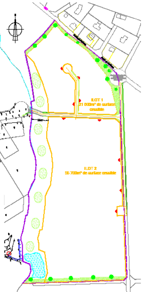
Plan d'aménagement
